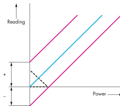
Fig. 42: Zero offset
